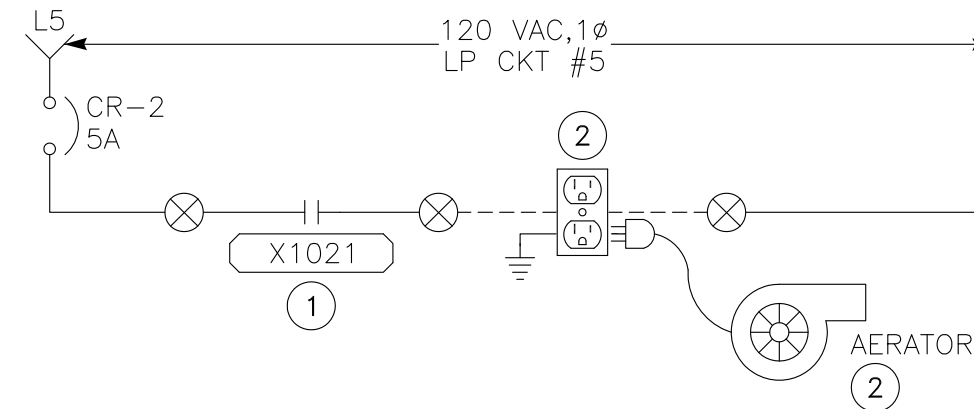
AERATOR CONTROL DIAGRAM (B) E10.6
